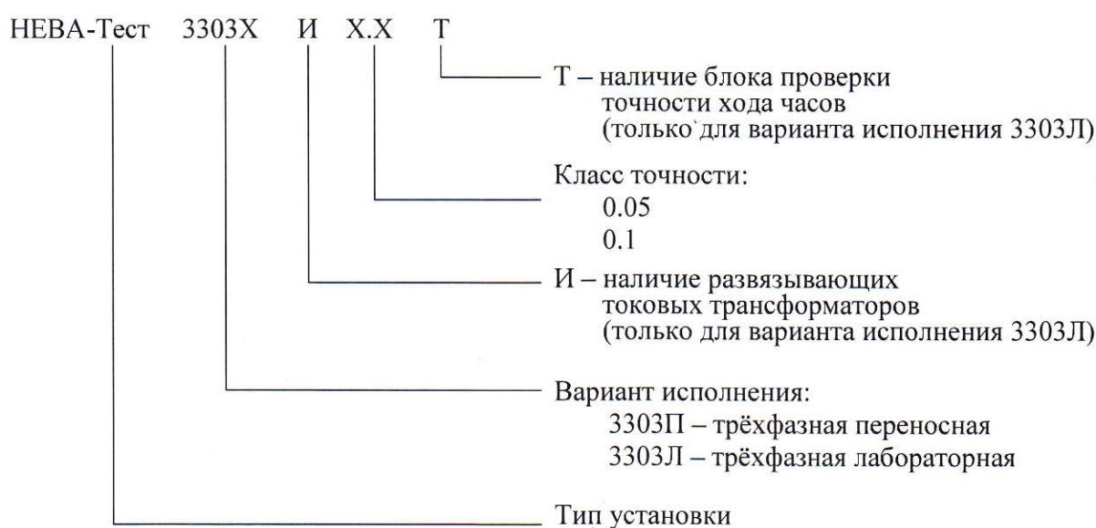
Рисунок 1 - Структура обозначений исполнений установок
